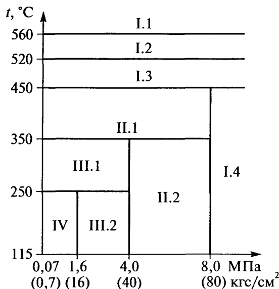
Схема зависимости категорий трубопроводов от значений параметров среды
